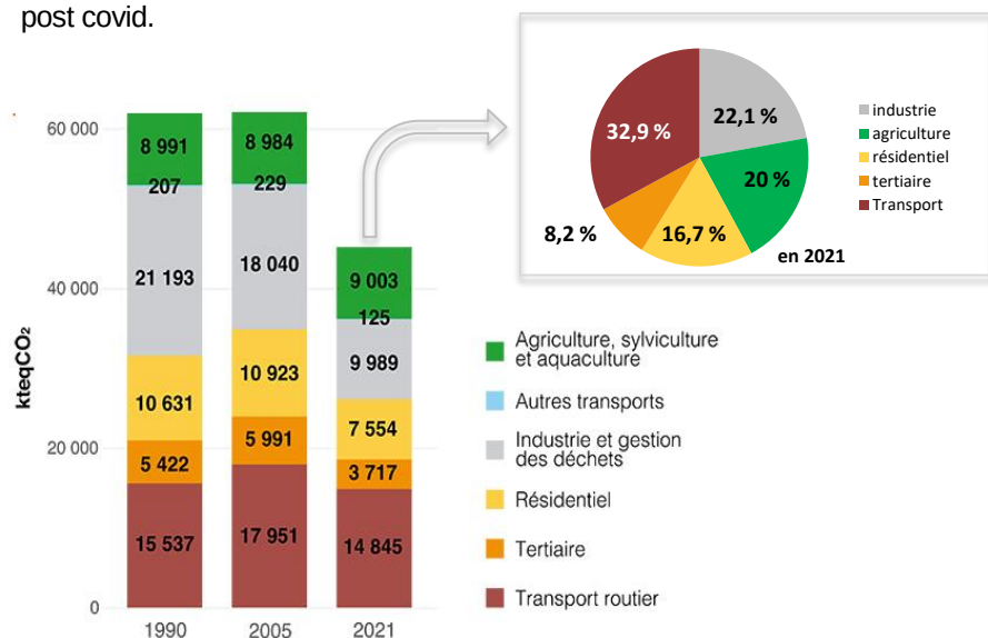
Évolution des émissions de GES (hors gaz fluorés) par secteur (1990-2005-2021) en kteqCO 2
