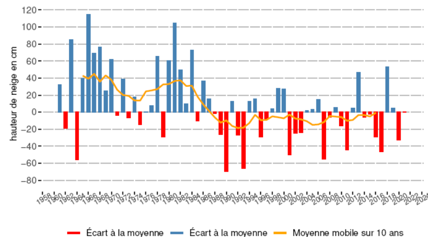
Evolution de l'écart à la moyenne 1960-2021 de la hauteur de neige moyenne au col de Porte (1325m)
