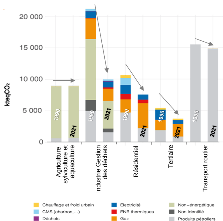
Comparaison des émissions de GES (hors gaz fluorés) par secteur et par énergie entre 1990 et 2021 (kEqCO 2 )
